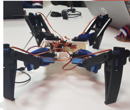
Робот-инспектор систем водоотведения ITквантум
